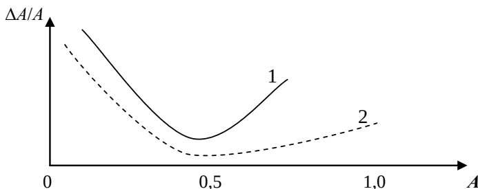
Рис. 6.21. Относительная погрешность измерений оптической плотности: 1 – теоретические расчеты; 2 – экспериментальные данные для некоторого спектрометра
