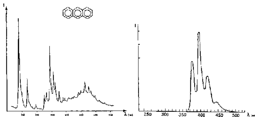
Рис. 6.29. Спектр люминесценции раствора антрацена в n -гексане при комнатной температуре (справа) и при -196\text{ }^{\circ}\text{C} (слева)
