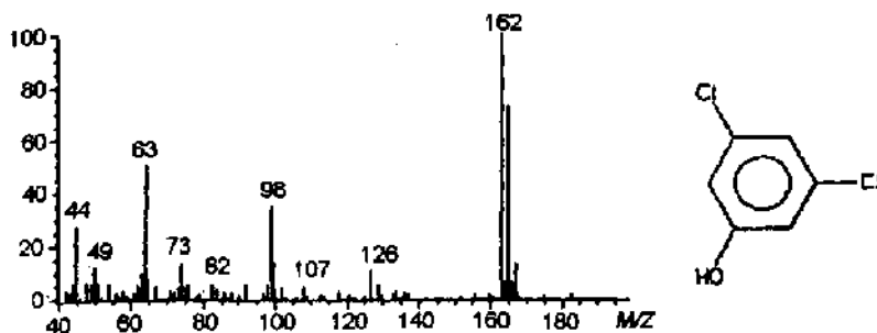
Рис. 6.31. Эталонный масс-спектр и структурная формула 3,5-дихлорфенола
